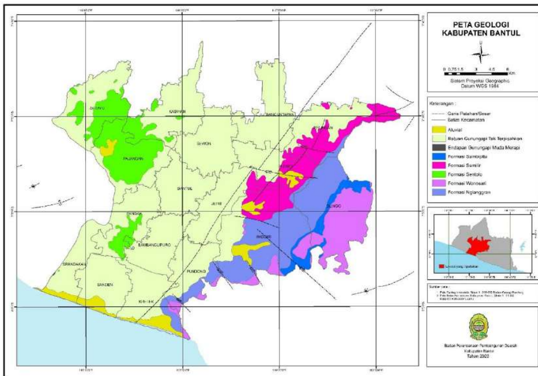
Gambar 2 5 Peta Geologi Kabupaten Bantul
